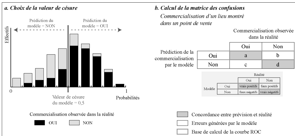
Figure 5. Principes généraux de la régression logistique binaire
