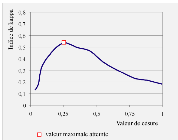
Figure 7 : Valeurs de l'indice de Kappa
