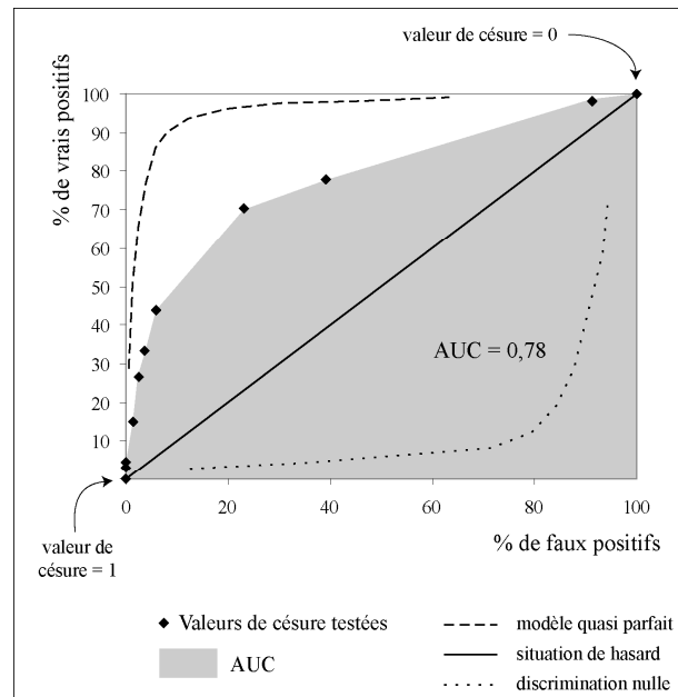
Figure 6 : Calcul de courbe ROC et de l'indicateur AUC
